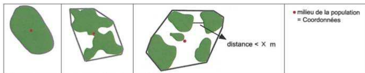
Fig. 6 : représentation schématique d'une aire de présence (source: RACFAA)
